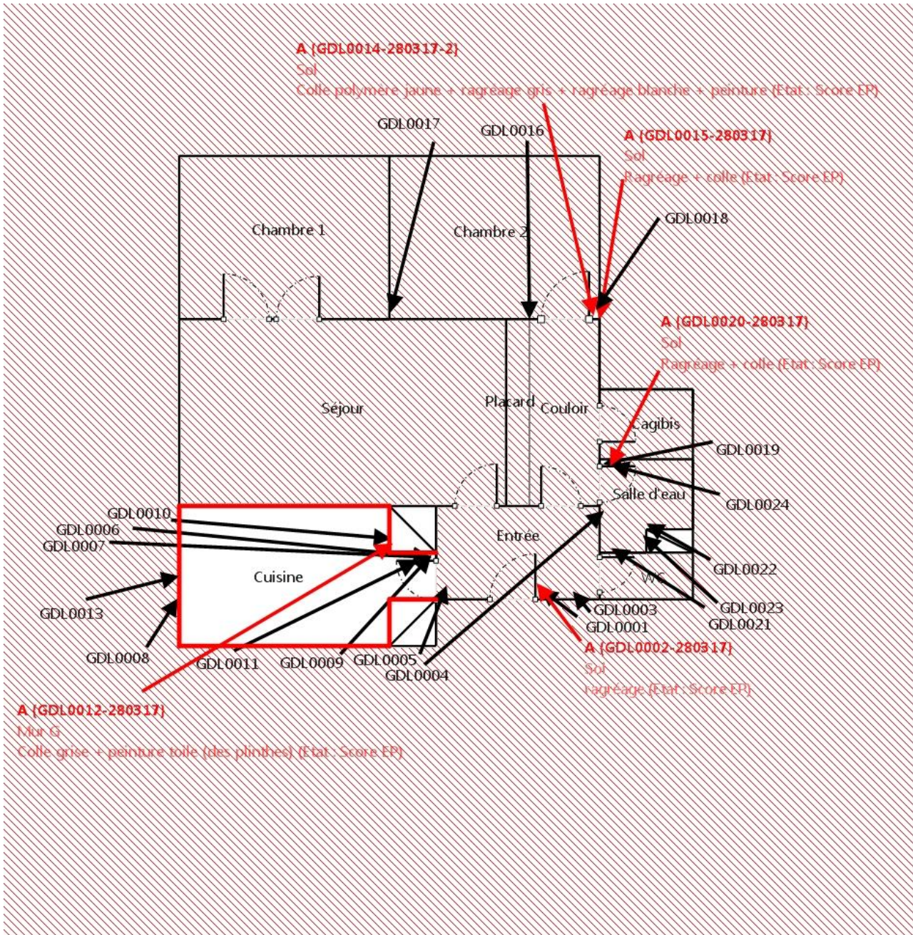
Planche (croquis) de repérage technique effectué par le cabinet : ALLODIAGNOSTIC, auteur : Geraud DE LAFFON Dossier n° 860459 du 28/03/2017 Adresse du bien : 3 SQUARE PAUL ALGIS ESC AC 50LAC0103 (50LAC0103) 77360 VAIRES SUR MARNE
